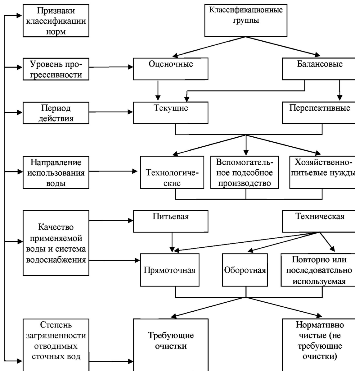
Рисунок 1 - Классификация норм водопотребления и водоотведения на ТЭС
