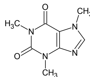
кофеин
