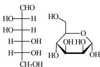
D -Манноза
