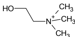
Холин
