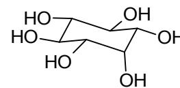
Инозит
