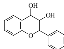
Флаван-3,4-диол
