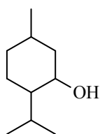
ментол
