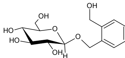
Салицин
