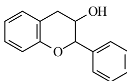
Флаван-3-ол
