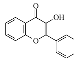
Флафон-3-ол
