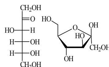
D -Фруктоза
