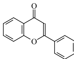
Флафон
