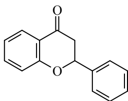
Флаванон
