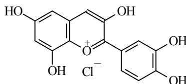
Цианидин
