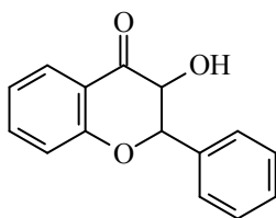
Флаванон-3-ол
