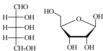
D -Рибоза
