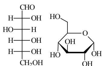
D -Глюкоза
