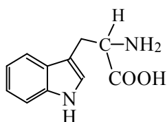
Триптофан ( Try )
