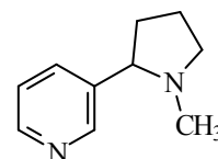
НИКОТИН
