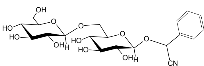
Амигдалин
