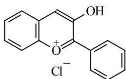
3-Гидрокси-2-фенилхромелийхлорид (антоцианидины)
