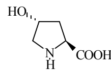
Гидроксипролин ( HyPro )
