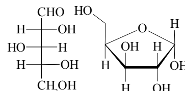
D -Ксилоза
