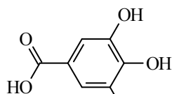
Галловая кислота
