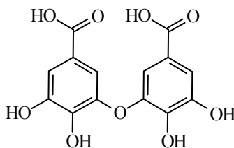
Дигалловая кислота
