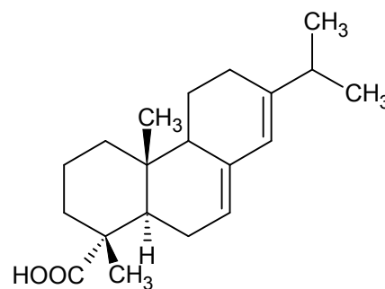
абиетиновая кислота
