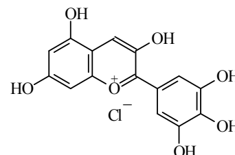
Дельфинидин
