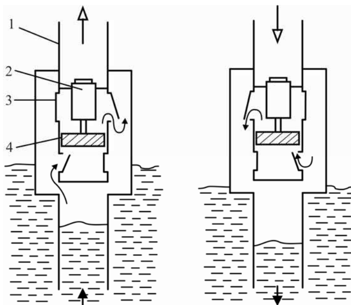
Рис. 9.13. Пневмобуй Масуды: 1 – корпус; 2 – электрогенератор; 3 – клапан; 4 – воздушная турбина
