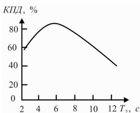
Рис. 9.10. Эффективность «утки Солтера» (диаметр 15 м, ось зафиксирована)
