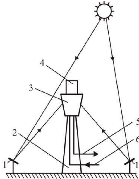
Рис 6.10. Схема СЭС:
