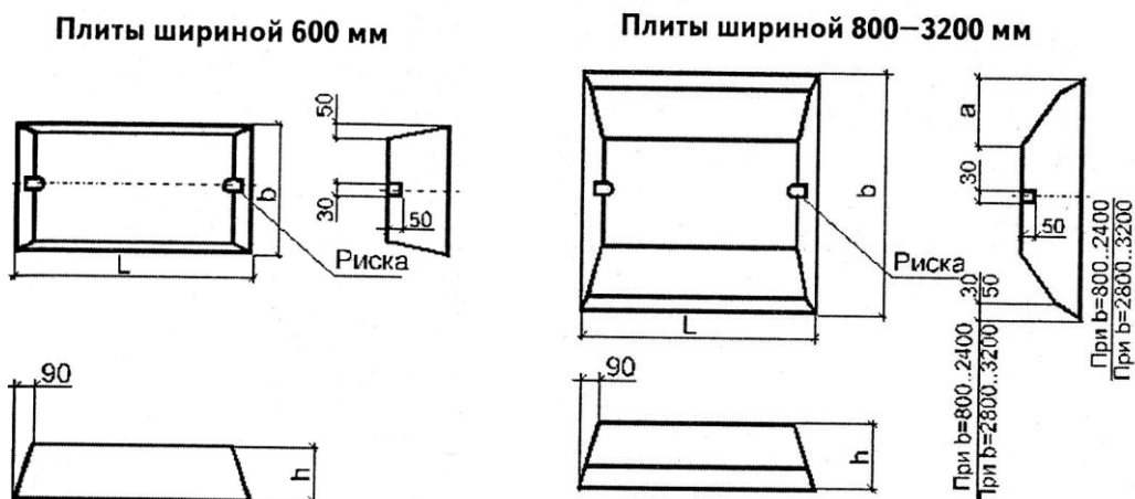
Рис. 2 Форма плит ленточных фундаментов
