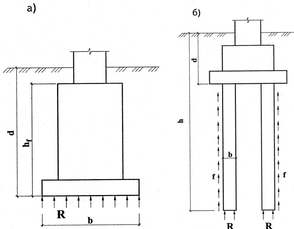
Рис. 1. Схемы фундаментов: а) мелкозаложенного; б) глубокозаложенного
