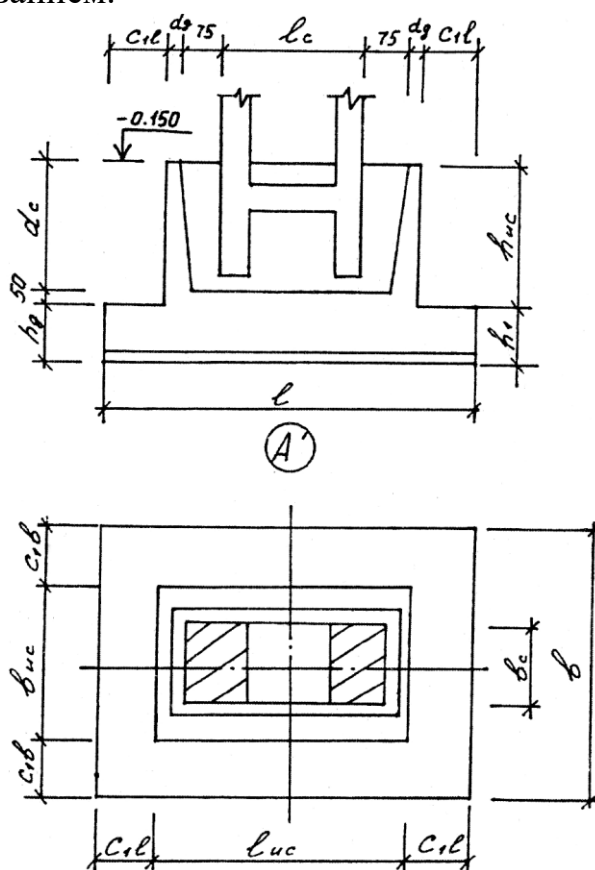
Рис. 3. Схема к формированию габаритов фундамента
